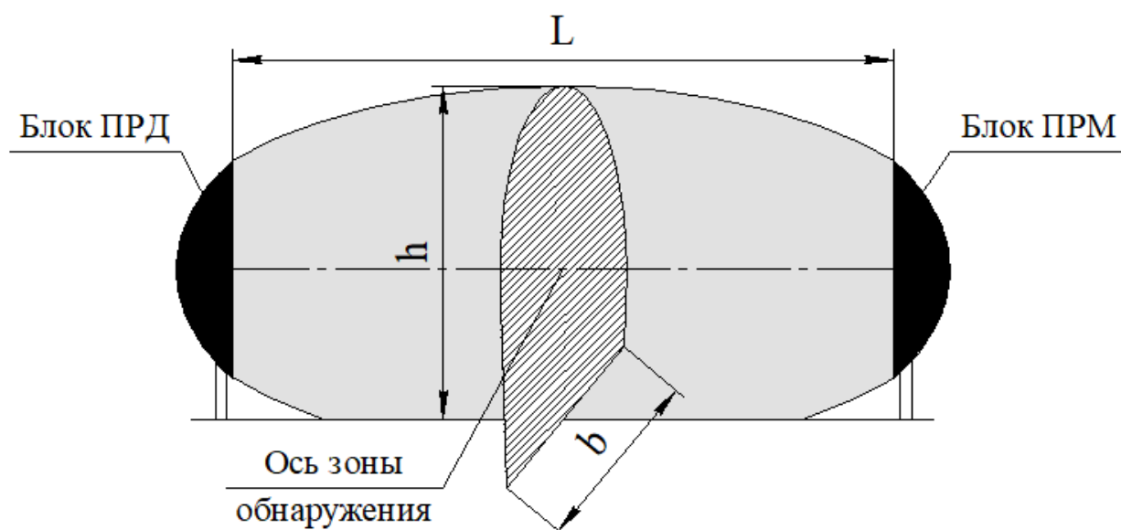
Рисунок 1.2 – Конфигурация зоны обнаружения, формируемой извещателями «ФОРТЕЗА-300-Ethernet», «ФОРТЕЗА-500-Ethernet»
